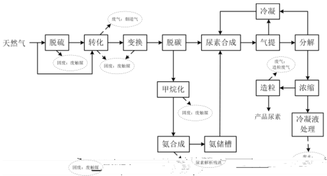
图 4-1 合成氨-尿素工艺流程图
